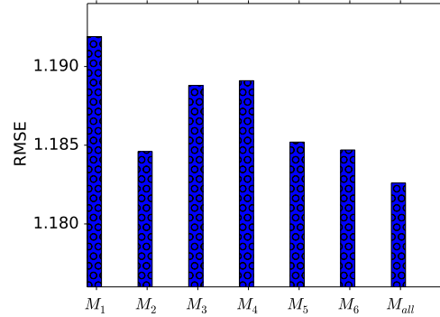
(b) Amazon.
